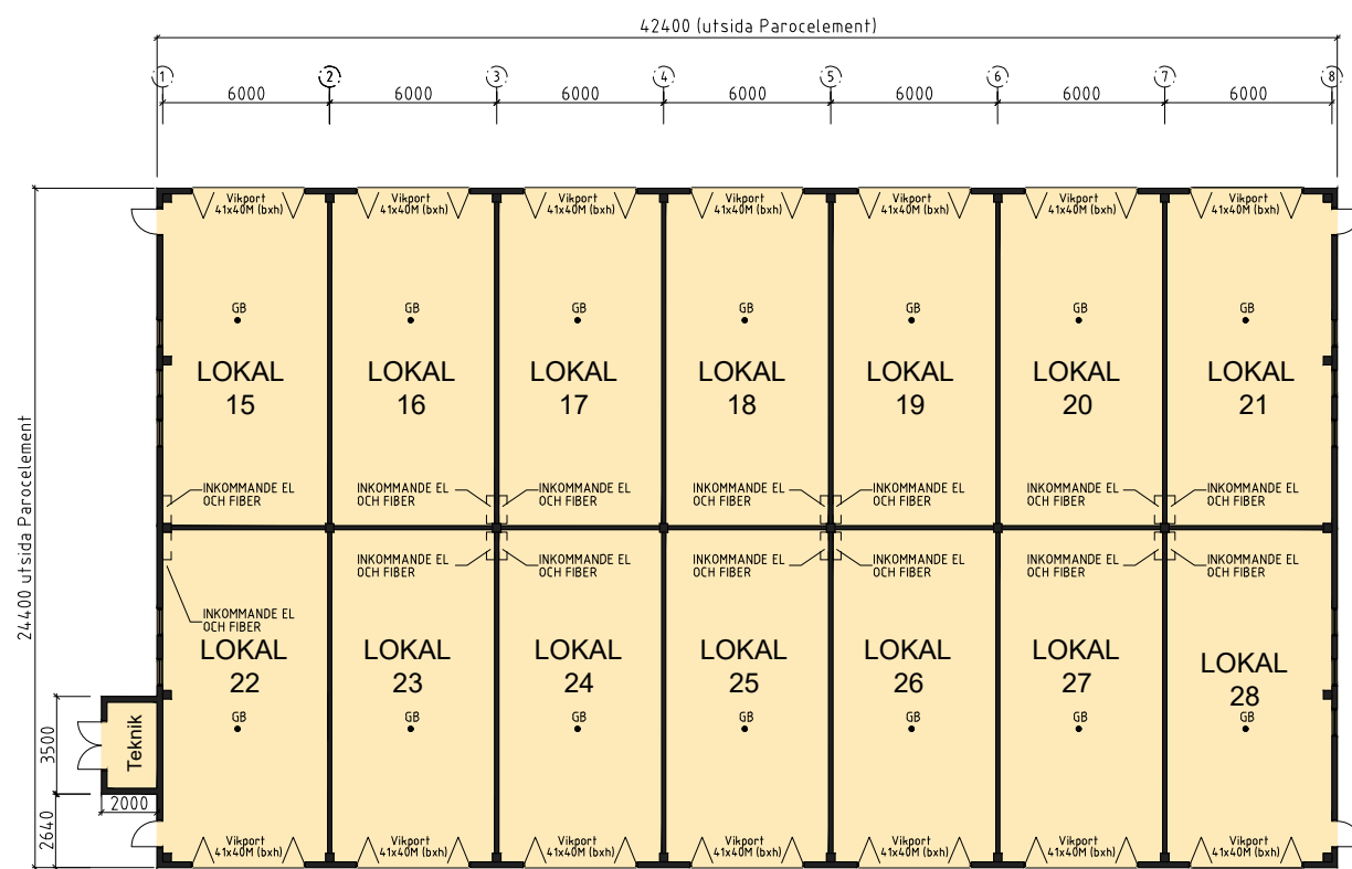
PLAN BOTTENVÅNING (HUS B) ←
