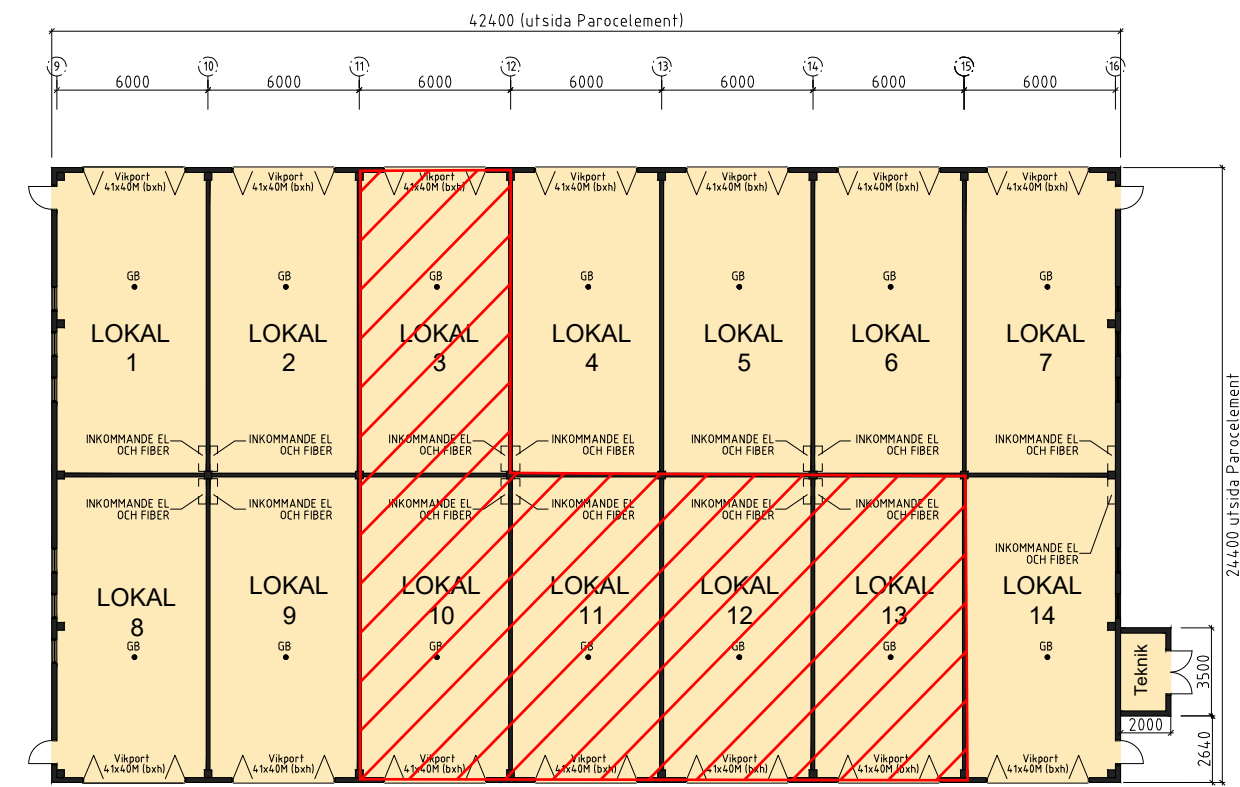
PLAN BOTTENVÅNING (HUS A) ←
