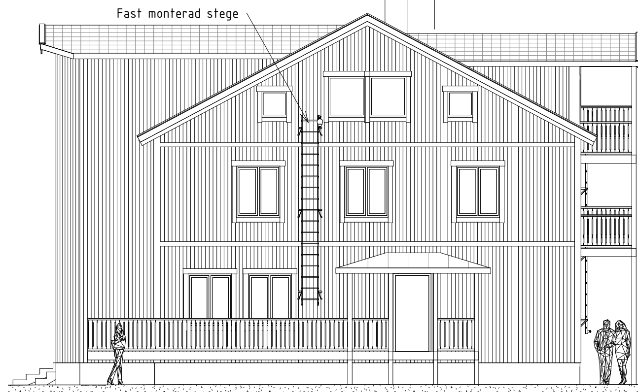
Fasad mot Sydöst
